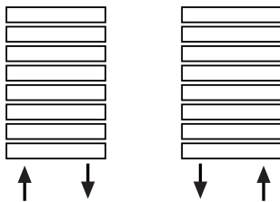
E ALLACCIAMENTO SCALDASALVIETTE CLASSIC-AL BATH CLASSIC-AL BATH towel warmer connection
