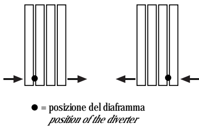
C ALLACCIAMENTO DAL BASSO CON DIAFRAMMA bottom connection with diverter
