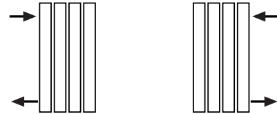
B ALLACCIAMENTO LATERALE side connection
